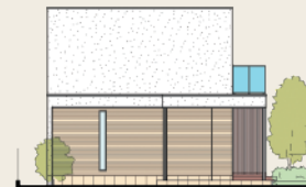
西立面図
